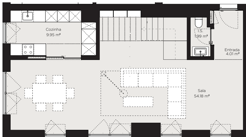
PISO 1
