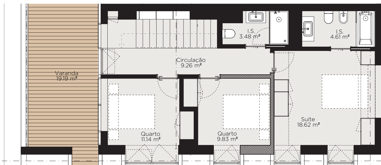
PISO 2
